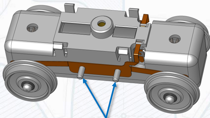
2 pions de fixation de chaque côté
