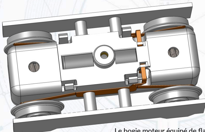
Le bogie moteur équipé de flancs de bogie
