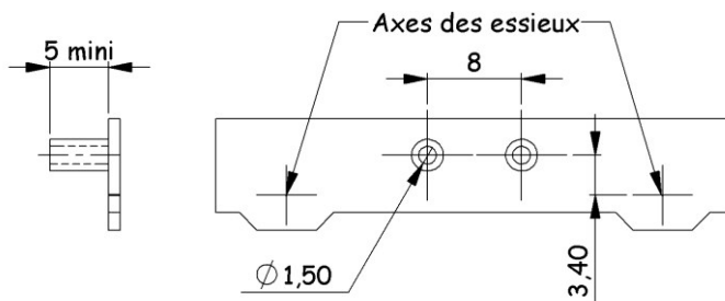
Dimensions et position des cylindres de fixation
